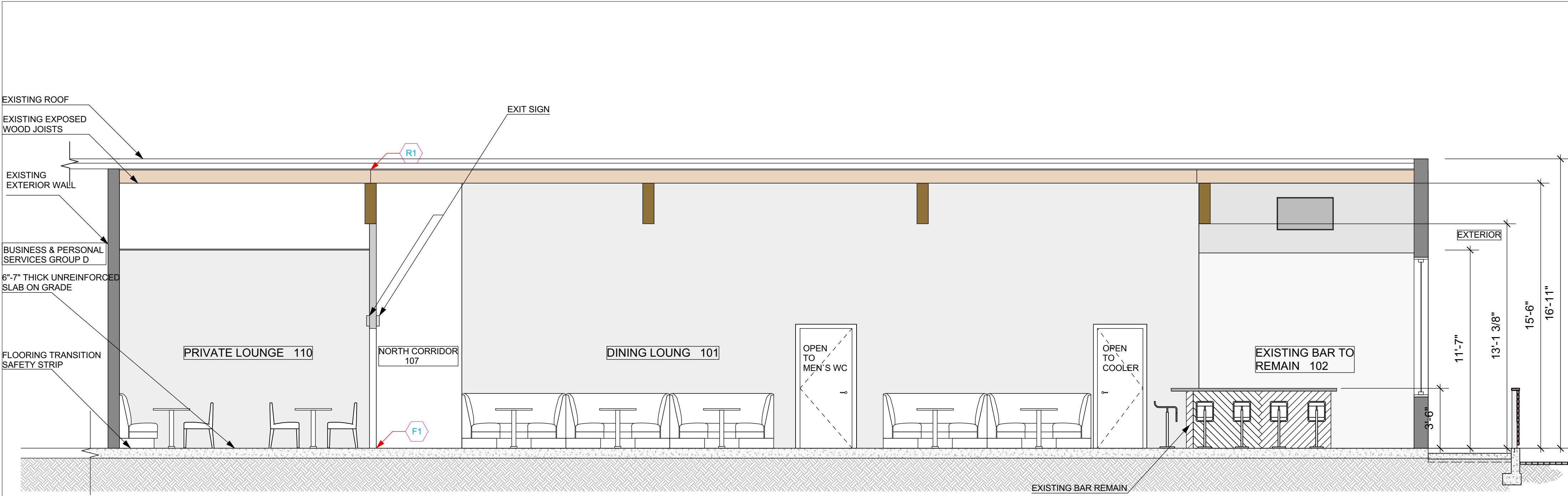
2 LONGITUDINAL SECTION VIEW EAST SCALE: 1/4" = 1'-0"
